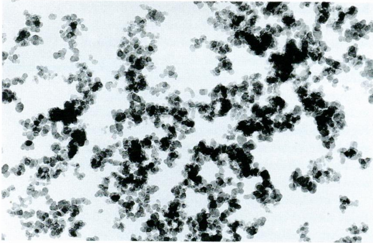
Abb. 11a: Furnaceruß mit hoher Struktur
